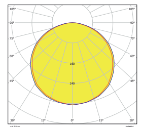
Vert Reticula Led 265 90 W OP
