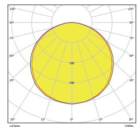
Vert Box Light 265 90 W OP
