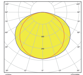
Vert Box Light 192 75W OP
