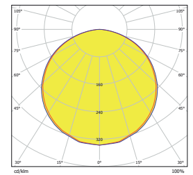
Vert Box Light 144 56W OP
